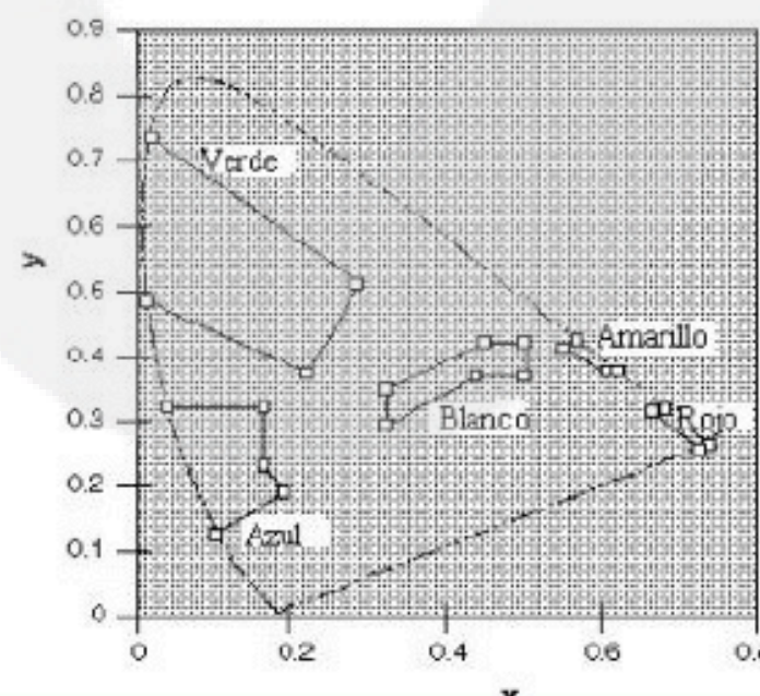
Figura 2: "Gráfico de Cromaticidad CIE1931"
